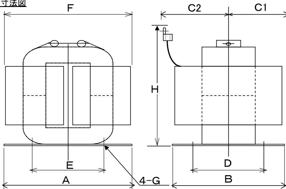
外形寸法図
